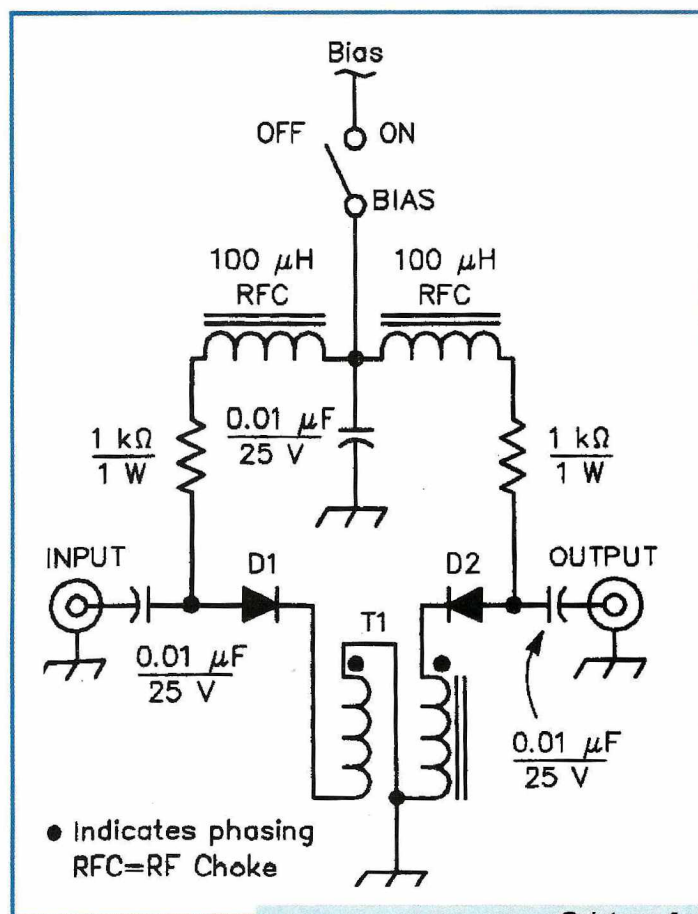
Schéma 4 : Essai de diodes.
