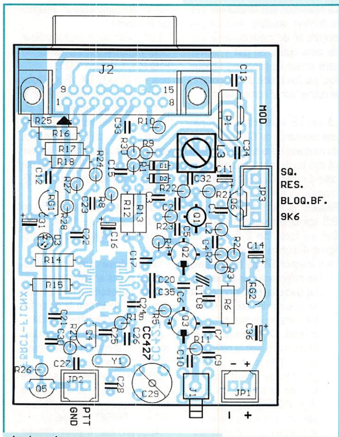
Implantation des composants.
