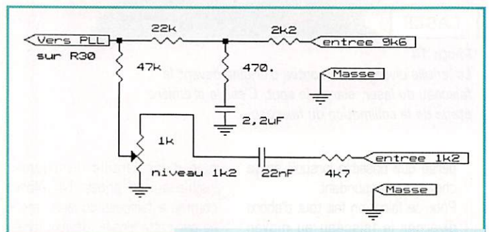
Figure 3 : Circuit externe pour le packet.
