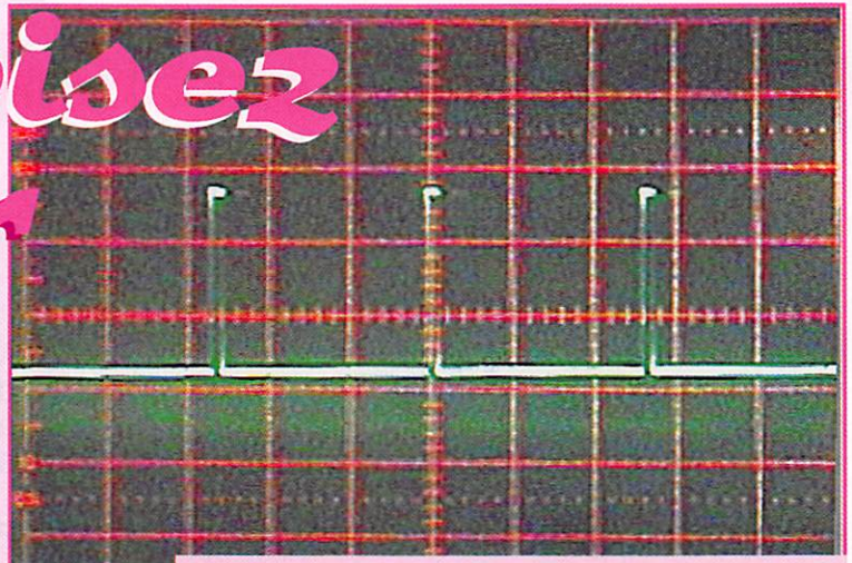
Photo 8 : En envoyant des impulsions brèves dans le primaire du transfo, on envoie un minimum de puissance au laser, ce qui permet un démarrage en douceur.
