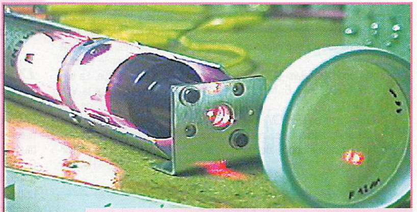
Photo 15 : La seconde étape du collimateur. Une lentille convergente, placée après la lentille divergente sur le trajet du faisceau, permet, en ajustant précisément l'espace entre les deux lentilles, de focaliser le spot à l'infini de manière à ce qu'il soit le plus net possible.
