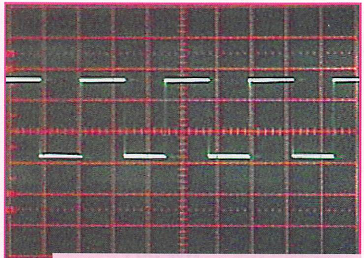
Photo 9 : Le maximum de puissance envoyée au transfo par le hacheur correspond à un rapport cyclique 1:1.
