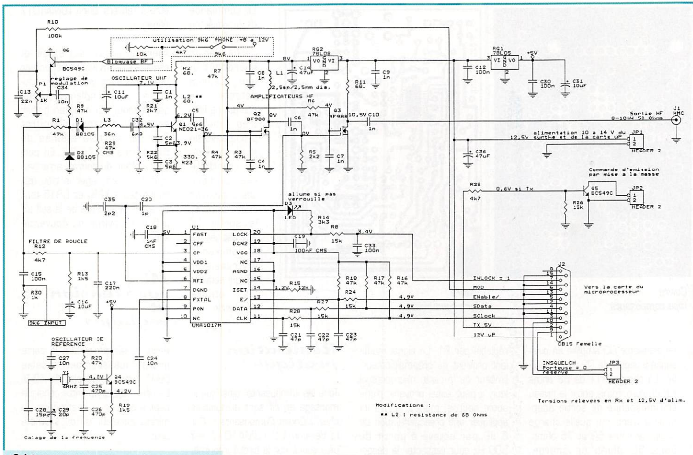
Schéma du synthétiseur UHF.
