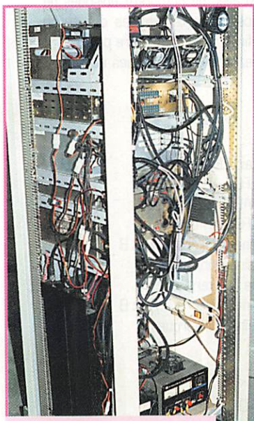
Vue arrière du relais : alims, duplexeur + filtres, ventilios, coaxiaux.
