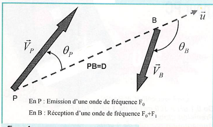
Figure 1 : Effet Doppler-Fizeau.
