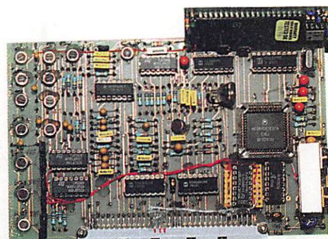
Carte logique principale : gestion relais PTT, CTCSS, BF, 1750.
