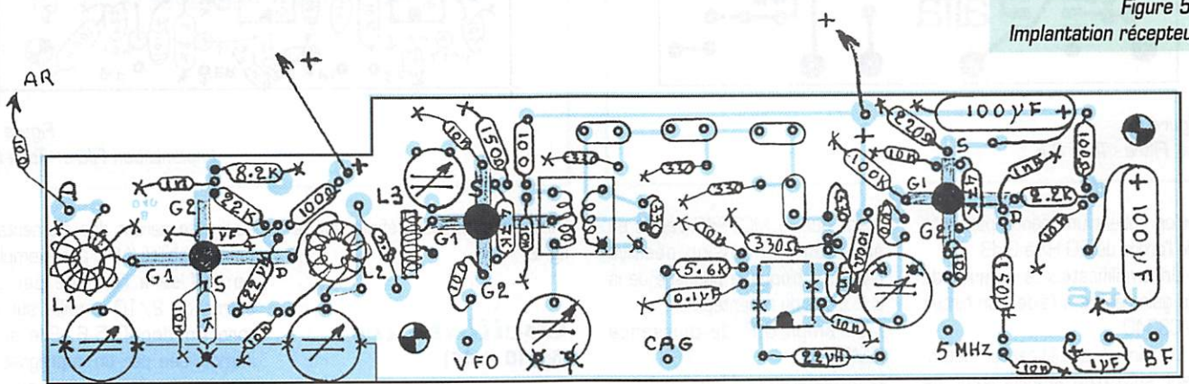
Figure 4 : C.I. Récepteur.
