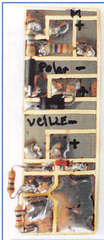
Platine de sécurité vue côté soudures et composants. Le thyristor n'est soudé que lorsque cette platine est mise en place.
