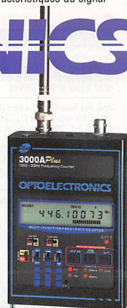
3000A-Plus Fréquence portable. 10 Hz à 3 GHz. Mémoire des 3 dernières mesures. Interface ordinateur
