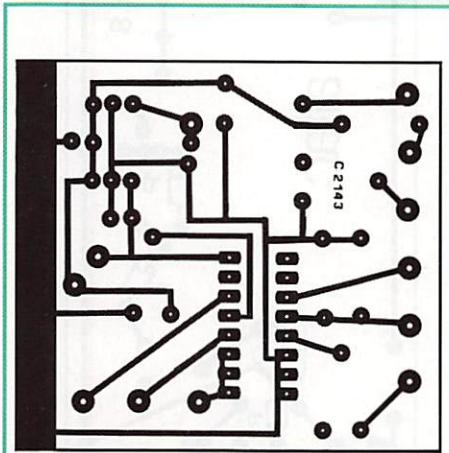
Figure 19 : C.I. Auxiliaires.
