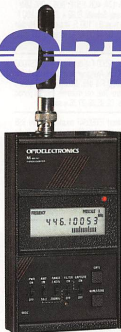
M-1 Fréquence portable. 20 Hz à 2,8 GHz
