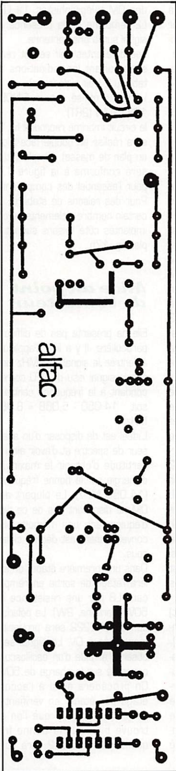
Figure 16 : C.I. Emetteur.
