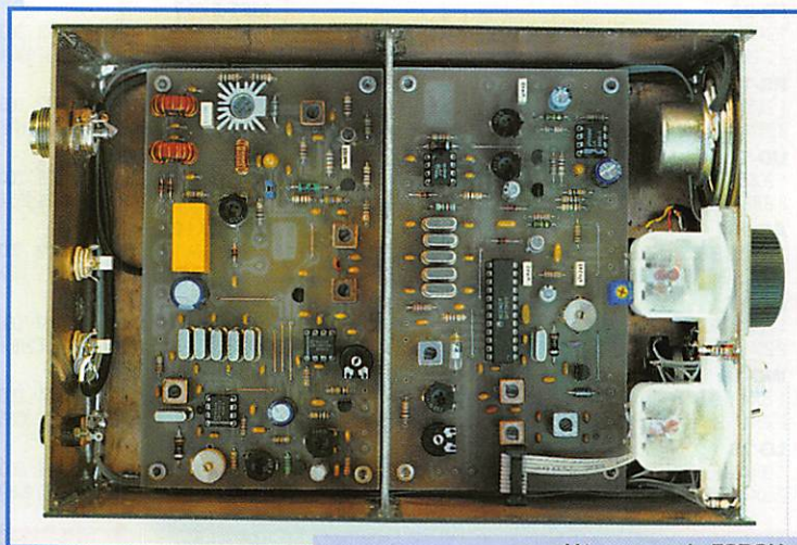
L'émetteur de F6BQU déjà décrit dans MEGAHERTZ.
