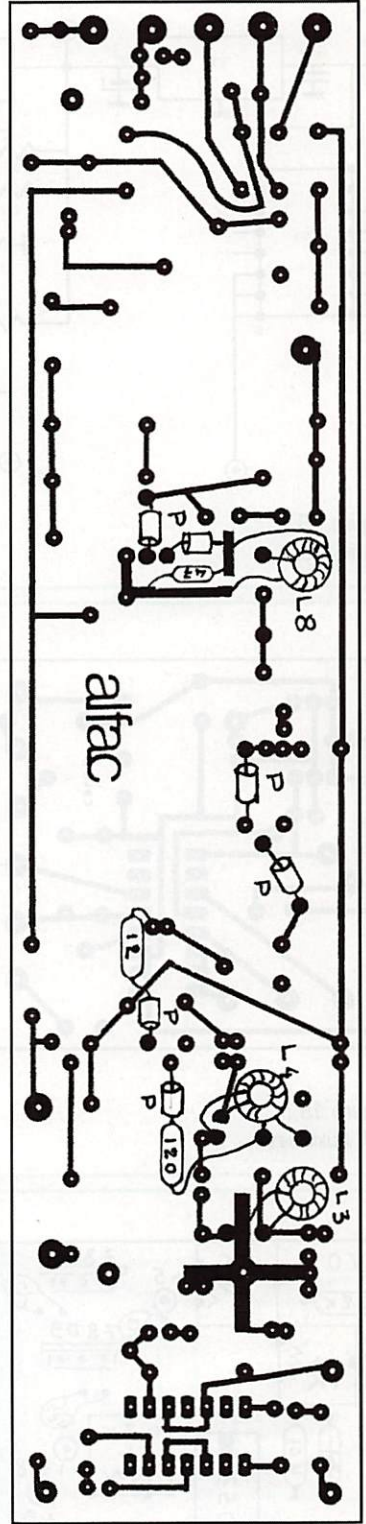
Figure 17b : Implantation Emetteur.
