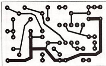
Platine imprimée supportant le circuit de la figure 1 ainsi que la variante de la figure 2.
