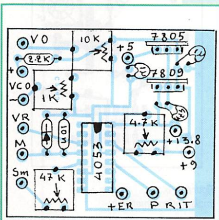
Figure 20 : Implantation Auxiliaires.
