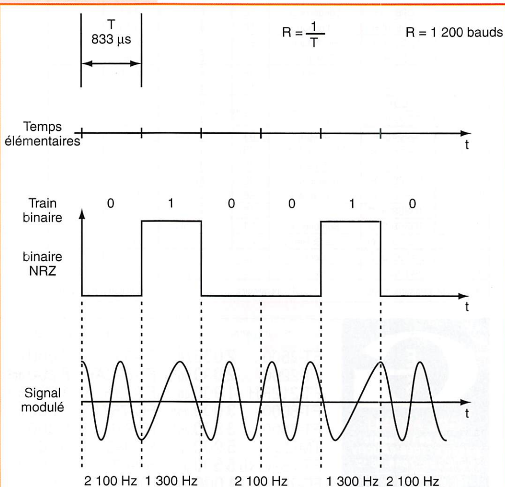
Figure 1 : Modulation Avis V23 intervalle de temps.
