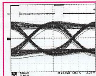
Diagramme de l'œil avec amplification des fréquences hautes.
