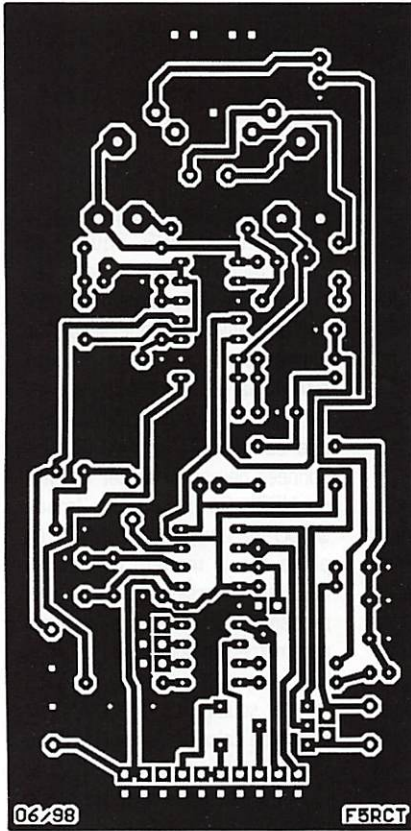
Circuit imprimé face soudures.
