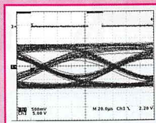
Diagramme de l'œil avec atténuation des fréquences hautes.
