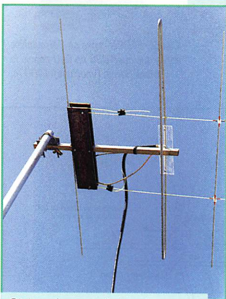
Côté trombone : on distingue les plaquettes de bois servant à maintenir l'écartement des fils nylon, ainsi que la boucle de symétrisation en RG142.
