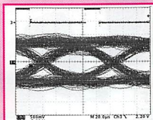
Diagramme de l'œil avec du bruit.
