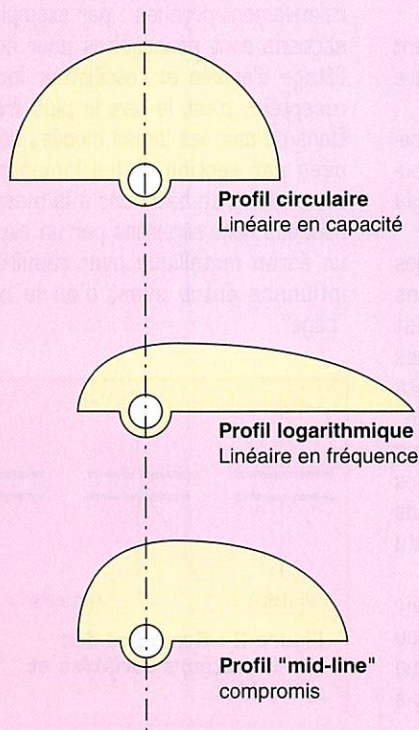
Figure 4 : Les divers profils des lames mobiles d'un CV.
