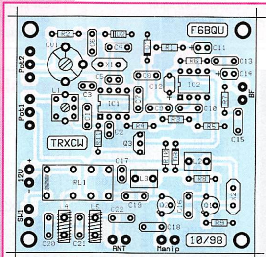
Implantation du TRX 80 m CW.
