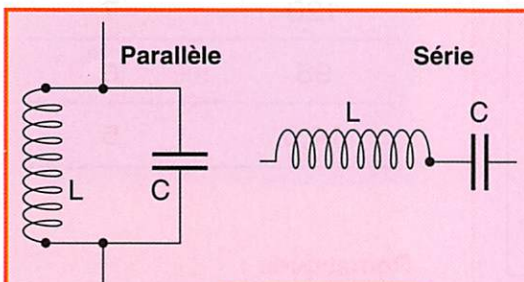
Figure 1 : Association de L et C en parallèle et en série.
