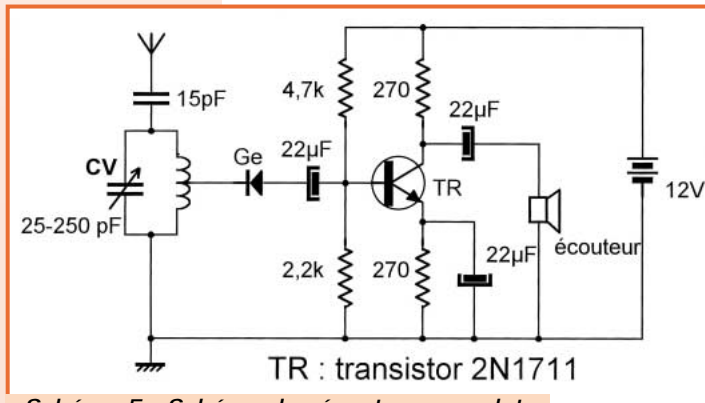
Schéma 5 - Schéma du récepteur complet.
