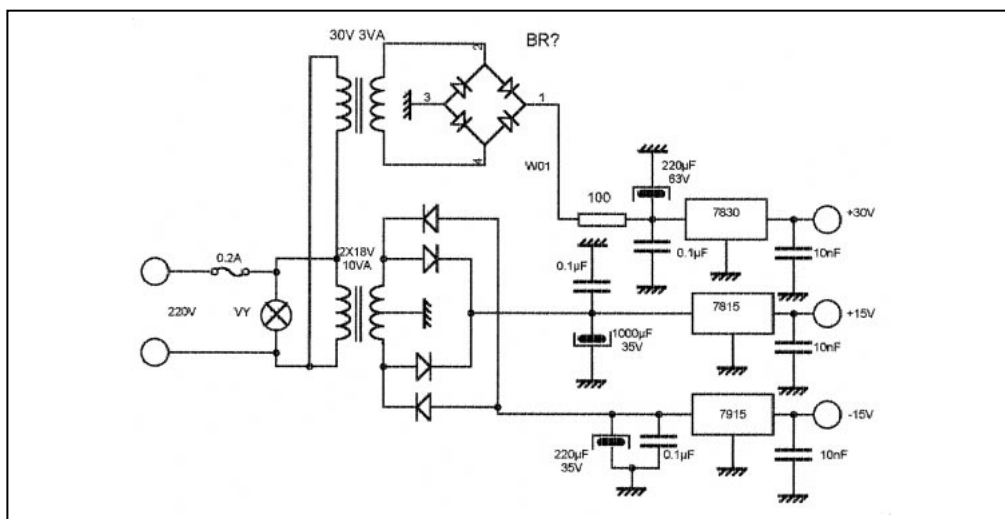
Synoptique.3 Wobulateur 0,5-45 MHz.
