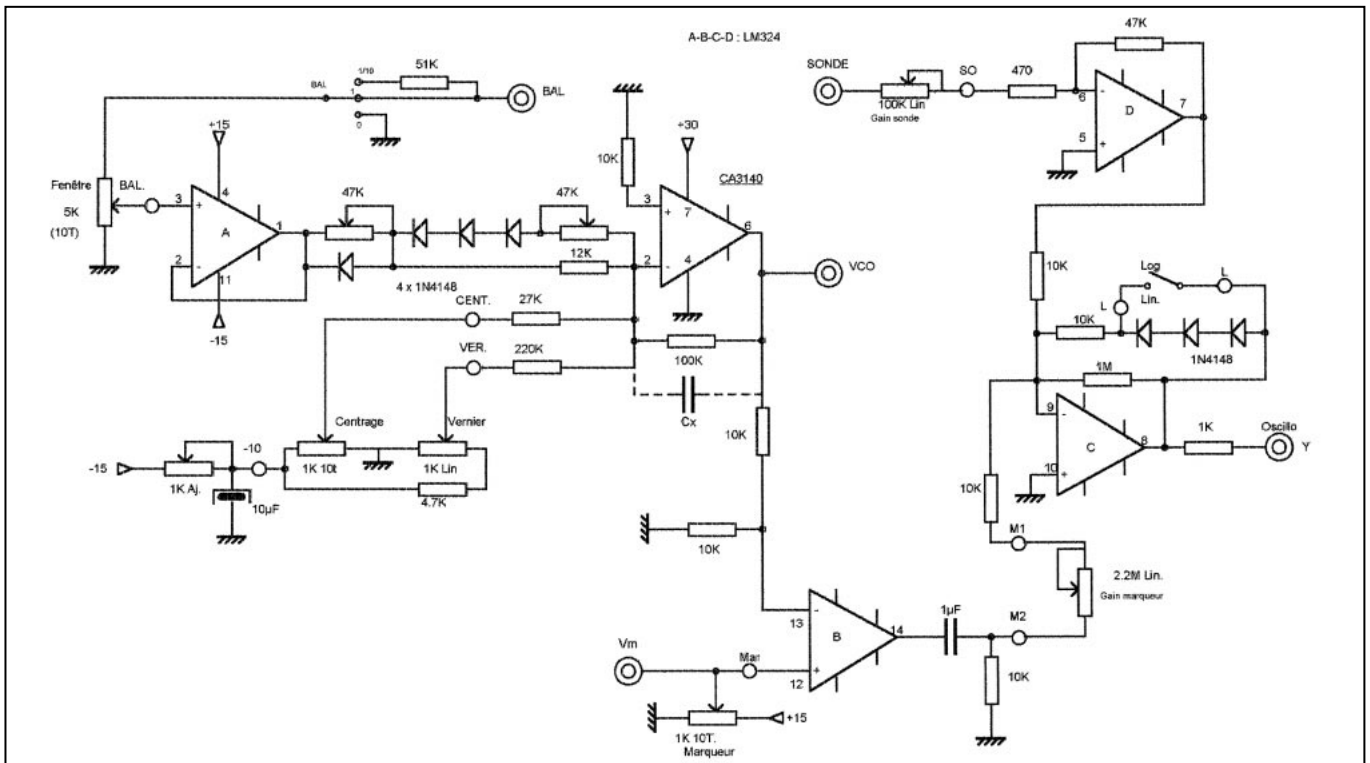
Synoptique.2 Wobulateur 0,5-45 MHz.
