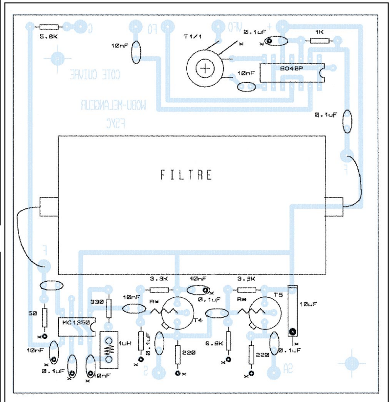
Implantation.4 Wobulateur 0,5-45 MHz.
