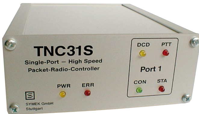
Le TNC31S, contrôleur packet 16 bits avec modem 153600 bauds.
