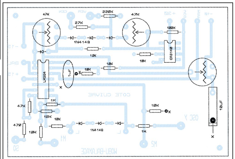
Implantation.5 Wobulateur 0,5-45 MHz.
