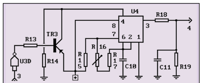
Figure 3 - Oscillateur.
