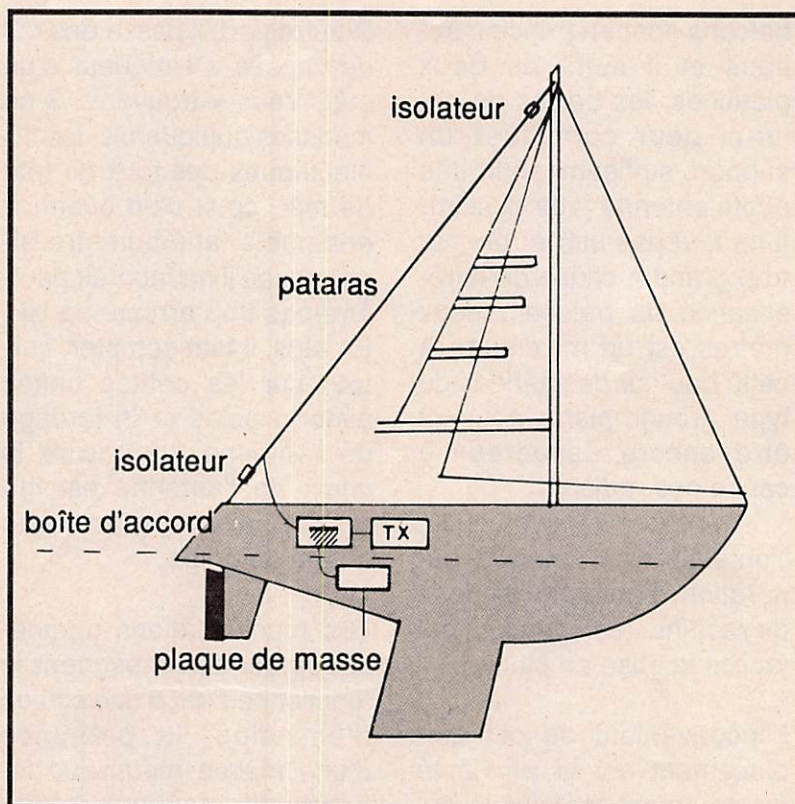
Plaques de masse : plaque de bronze de faibles dimensions (≈ 30 cm x 20 cm) placée sous la flottaison et dont la surface est constituée de fines billes de façon à offrir une grande surface de contact.
