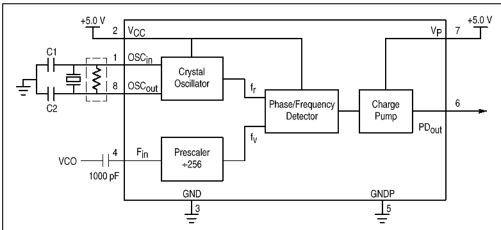
Figure 14 - Un synthétiseur simple avec le CI MC12179.
