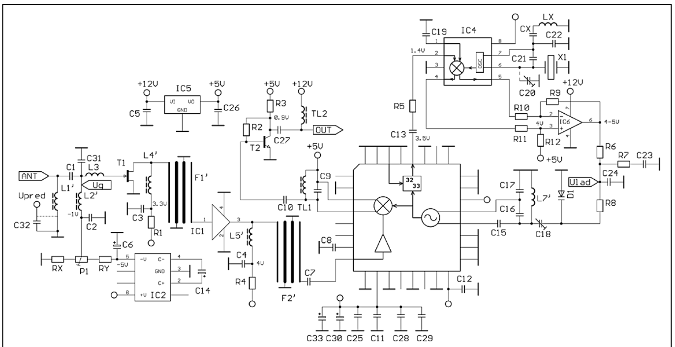
Figure 4 - Schéma du convertisseur.
