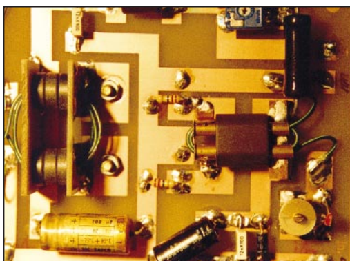
▲ Transformateur 1.
