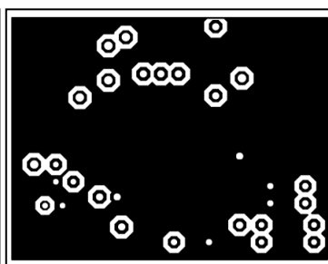
Figure 18 - Mylar du CI (dessous).
