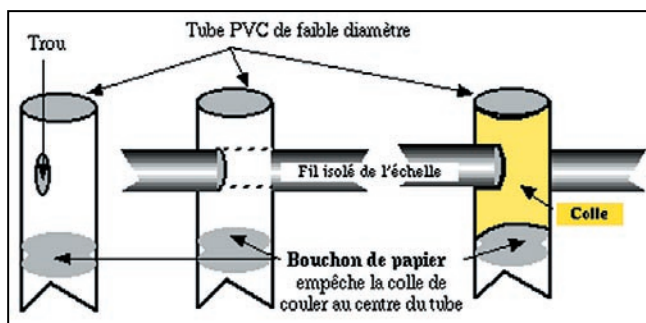
Figure L07 - Ecarteur de ligne d'alimentation en tube PVC.
