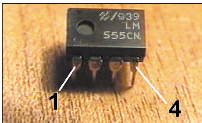
Photo 1 : Le circuit intégré 555 en boîtier DIL.
