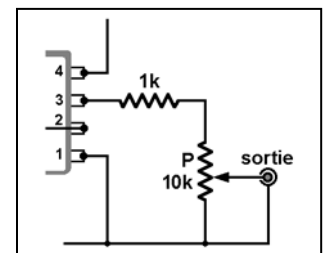
Figure 8 : Variante du circuit de sortie.
