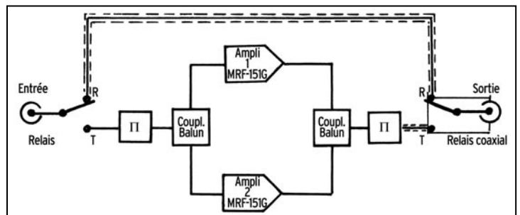
Figure 2 : Schéma synoptique de la partie HF.
