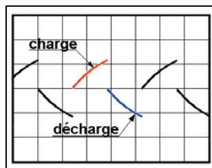
Figure 2: Représentation du signal observé sur la patte 6.
