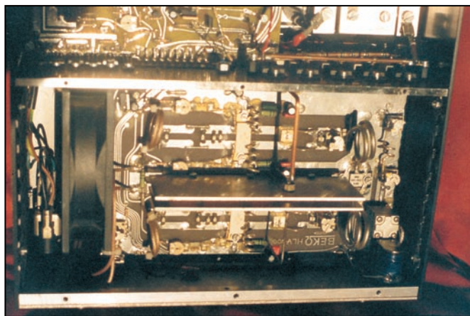
Photo 3 : Vue rapprochée du compartiment HF : on y distingue le ventilateur axial à gauche, les deux transistors TMOSFET au centre, le coupleur hybride et le relais coaxial de sortie à droite. La carte est directement fixée au dissipateur qui se trouve dessous.
