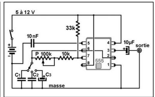
Figure 7 : Schéma du générateur BF à signaux carrés.
