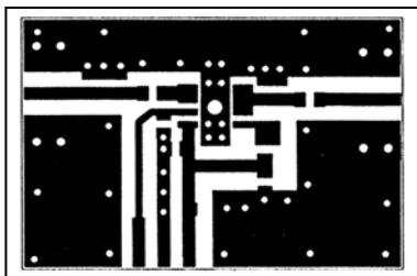
Circuit imprimé.
