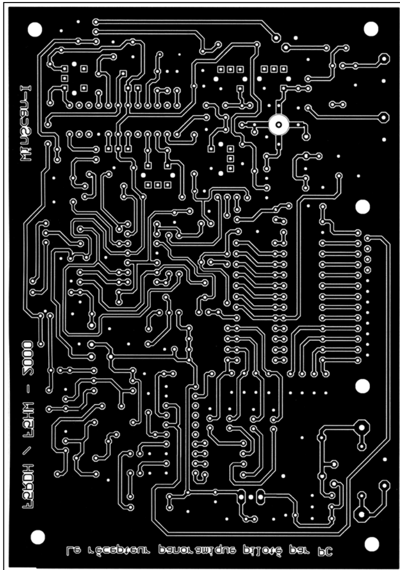
Circuit imprimé.
