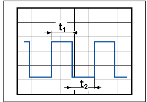
Figure 5 : Le signal carré et ses deux demi-périodes.
