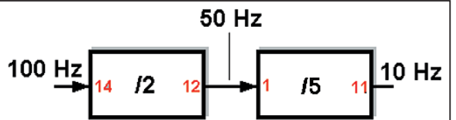
Figure 1 : Principe du 7490.
