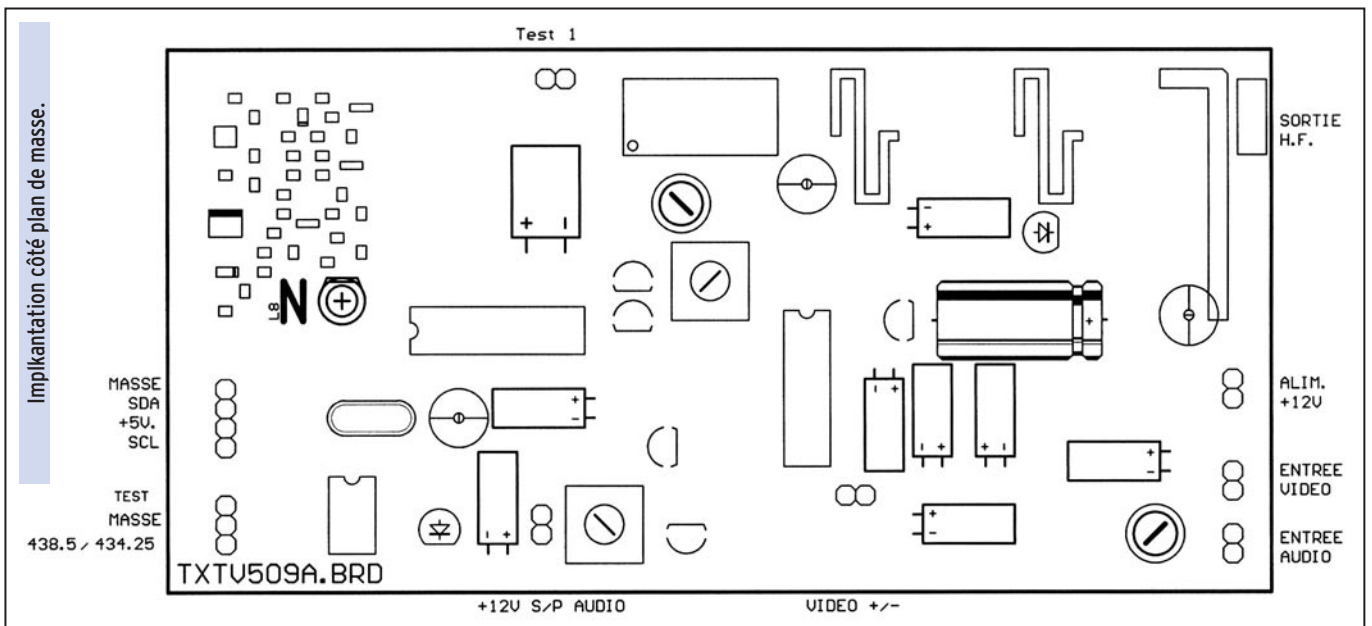
Circuit côté plan de masse.
