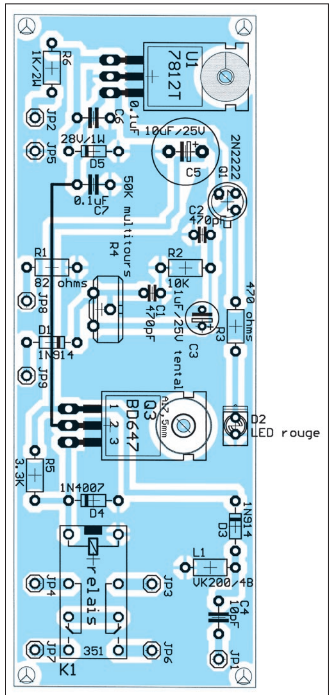
Figure 6 : Implantation des fonctions annexes.
