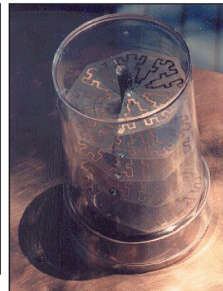
Figure 20 : Une antenne hélice miniaturisée grâce à la fractalisation. Nathan Cohen NIIR.
