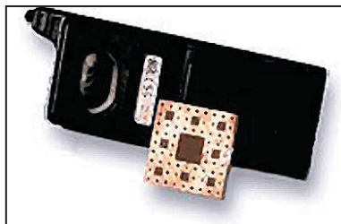
Figure 7 : Une antenne fractale en circuit imprimé, destinée à être montée à l'intérieur du téléphone portable. (Document communiqué par Nathan Cohen NIIR).
