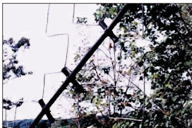
Figure 14 : Un des bras de l'antenne de N1IR avec les entretoises supportant les coudes de la boucle fractalisée.
