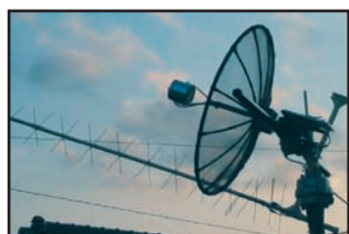
L'antenne du mois, celle de JF6BCC pour trafic via OSCAR 40.
