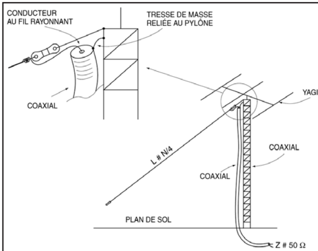
Figure 1 : Schéma de l'antenne Half Sloppler.
