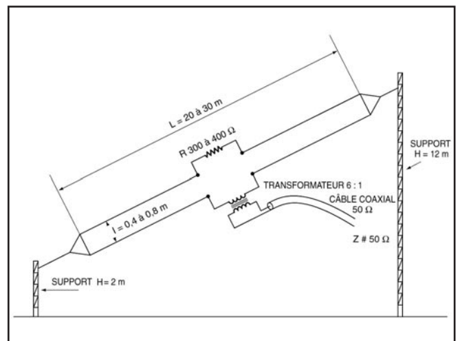
Figure 6 : Schéma classique de la T2FD.
