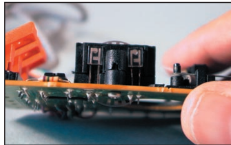
19 - Une souris disséquée : vue sur l'encodeur...
