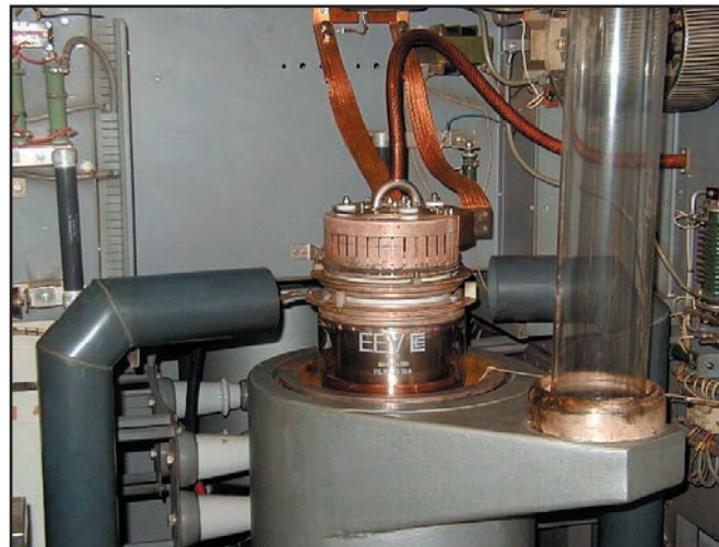
6 - Tube de l'étage de modulation
