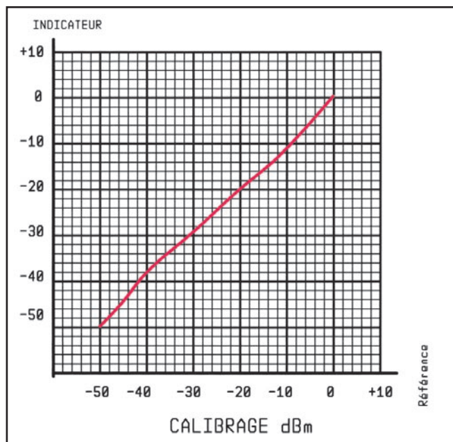
7 - Calibrage en dBm
