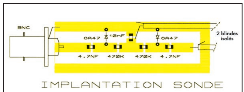
4 - L'implantation des composants
