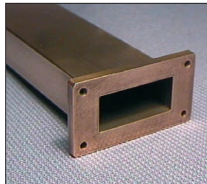
8 - Un guide d'onde pour les ondes centimétriques.
