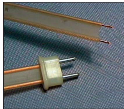
3 - Ligne bifilaire et la prise qui va avec.
