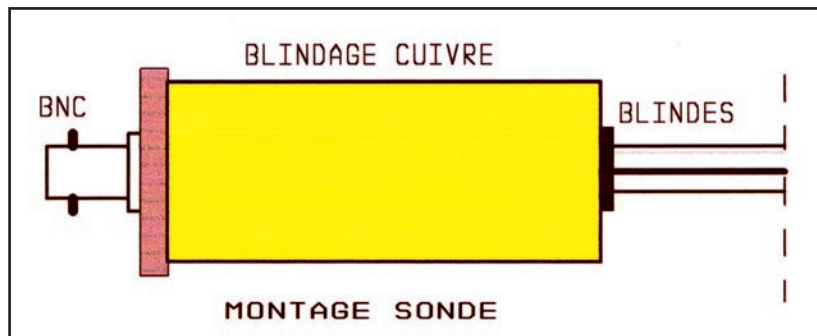
5 - Montage pratique dans un tube
