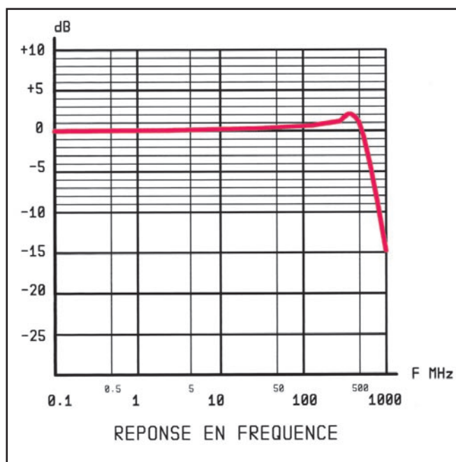
6 - Courbe de réponse en fréquence
