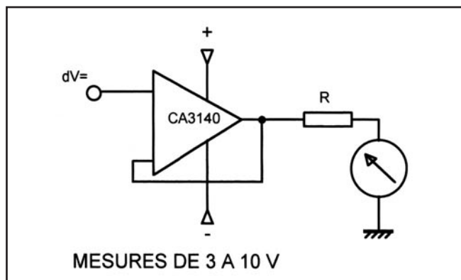
8 - Pour mesurer des tensions de 3 à 10 V
