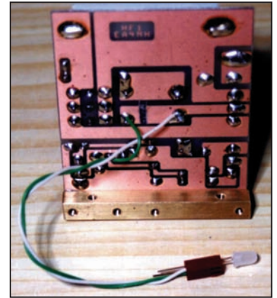
Figure 12 : Circuit du relais. Côté des soudures.
