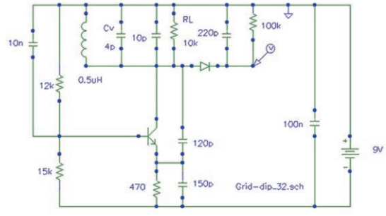
RI 1000k à 10K : Vdc va de 9.5 V à 8.8V ( avec 0.5uH , 4 pF à 21 MHz ) RI 1000k à 10K : Vdc va de 9.3V à 8.8V ( avec 0.5uH , 70pF à 17 MHz ) Spectre TRES sale , largeur de 0.7MHz à 50% d'amplitude @ 21 MHz
