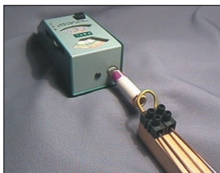
Photo 7: Le grid-dip couplé à la ligne.
