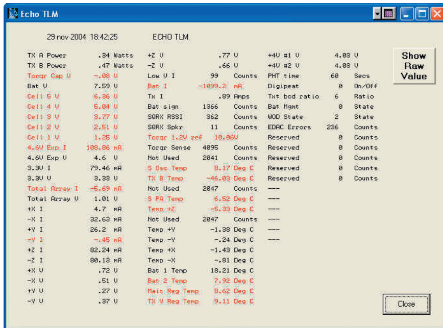
Figure 10: Télémétrie sous forme de texte.
