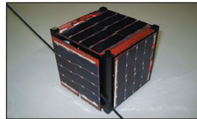
4 - Gros plan sur le microsattelite SEEDS-1
