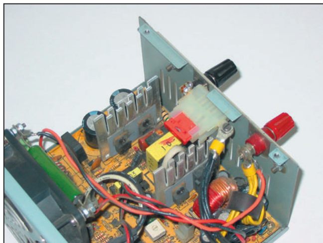
Photo 8: Par sécurité, un fusible a été installé en série avec la sortie. Lors des essais de mise au point, ce fusible était shunté et le débit permanent a été testé à 14 ampères pendant plusieurs heures.
