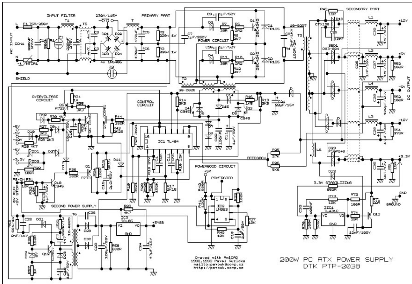
Figure 1: Schéma type d'une alimentation ATX pour PC de 200 W [4]. Même si votre alimentation diffère très légèrement, vous retrouvez en principe les mêmes éléments.
