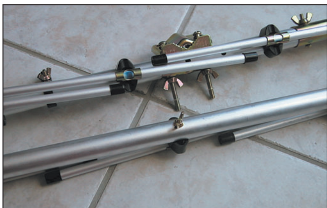
2 - Les éléments se replient le long du boom pour un transport facile.
