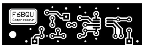
6 - Platine CI du compresseur.
