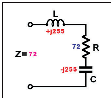
4 – Solution pratique pour que X_L et X_C s'annulent.
