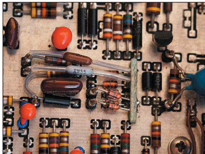
9 - Vue d'une modification SB pratiquée par Collins.
