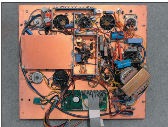
18 - L'envers du décor, le câblage du récepteur, à gauche l'étage HF sous le blindage.
