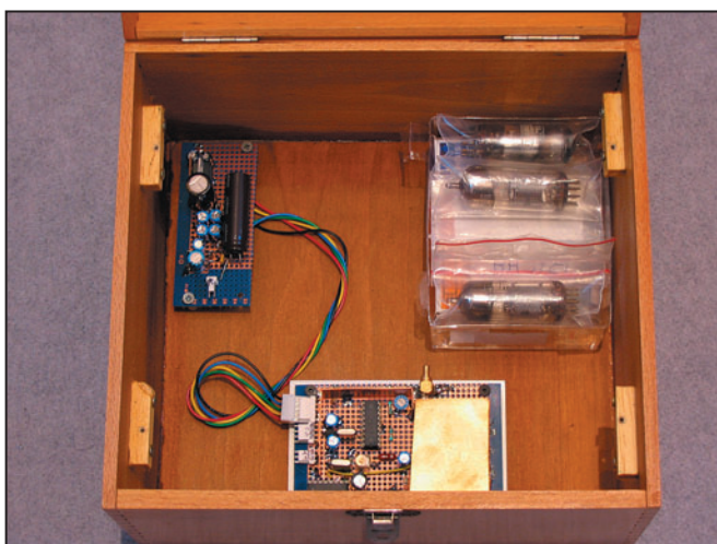
19 - Le fond du coffret avec l'alimentation continue, le synthétiseur et la réserve de tubes !
