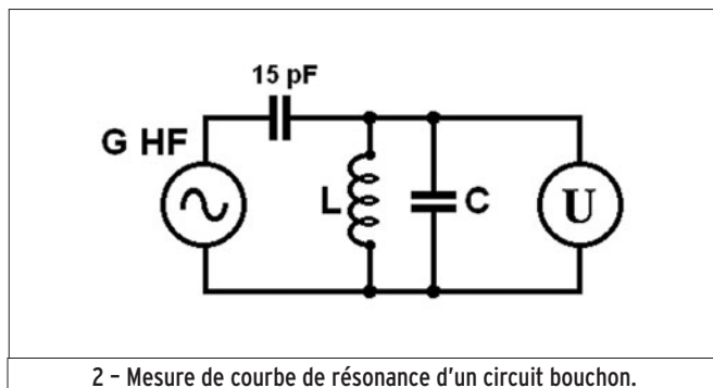
2 - Mesure de courbe de résonance d'un circuit bouchon.
