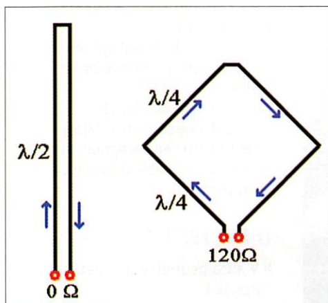
1 - De la ligne demi-onde à la boucle onde entière.
