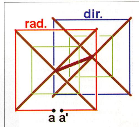
3 - Antenne cubical-quad à 2 éléments.
