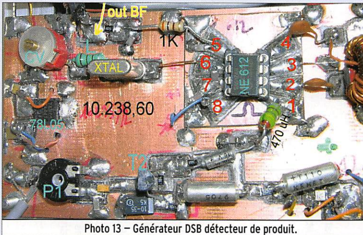
Photo 13 – Générateur DSB détecteur de produit.
