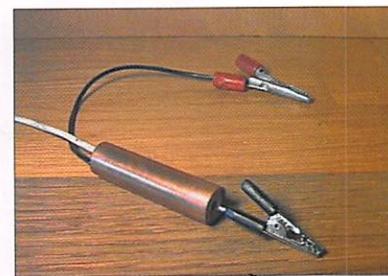
8 - Une sonde HF fabrication maison.
