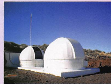
4 - L'observatoire SLOOH.
