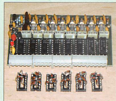
6 - AUX7 et 6 modules pour bandes WARC et broadcast.
