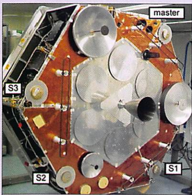
2 - Les antennes réception GPS sur AO-40.
