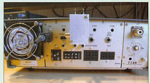
2 - TR-7 vue arrière avec le module atténuateur et coupleur hybride.
