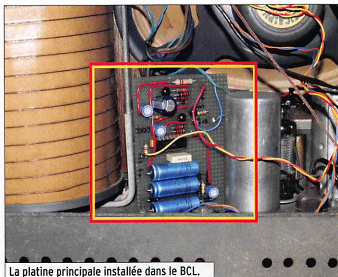
La platine principale installée dans le BCL.
