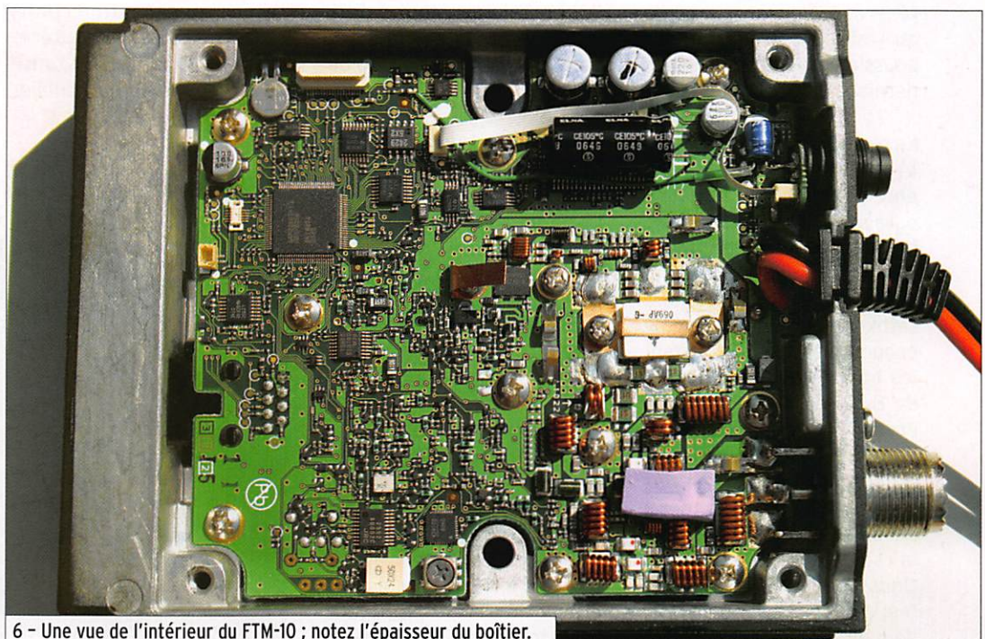
6 - Une vue de l'intérieur du FTM-10 ; notez l'épaisseur du boîtier.
