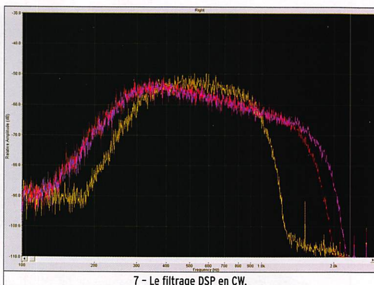
7 - Le filtrage DSP en CW.
