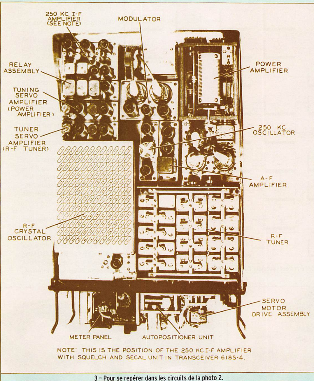
3 - Pour se repérer dans les circuits de la photo 2.
