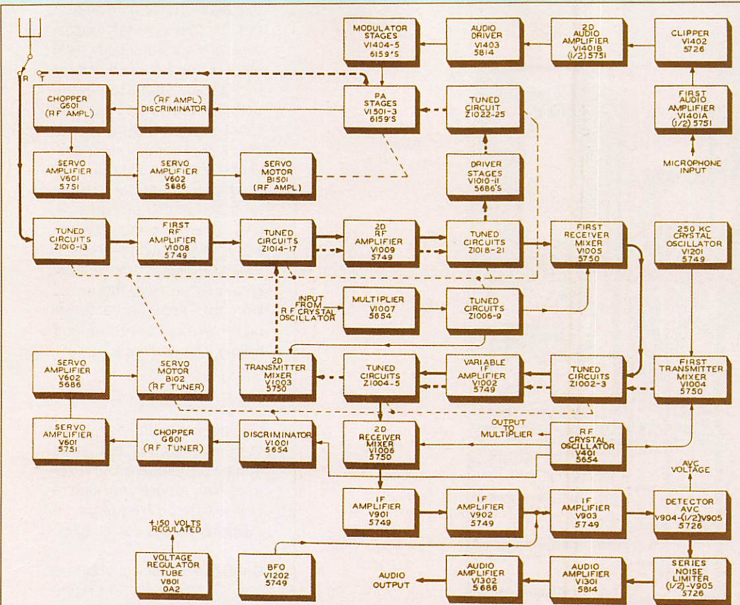
4 - Synoptique de l'émetteur-récepteur COLLINS 618S-1.
