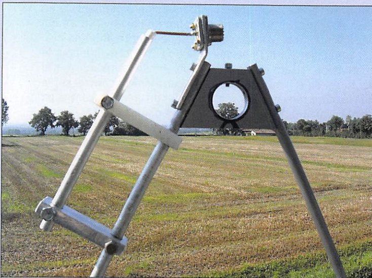
5 - Détail du gamma-match.
