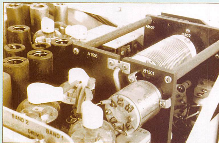
7 - Au premier plan le PA, au fond les 2 tubes du modulateur.
