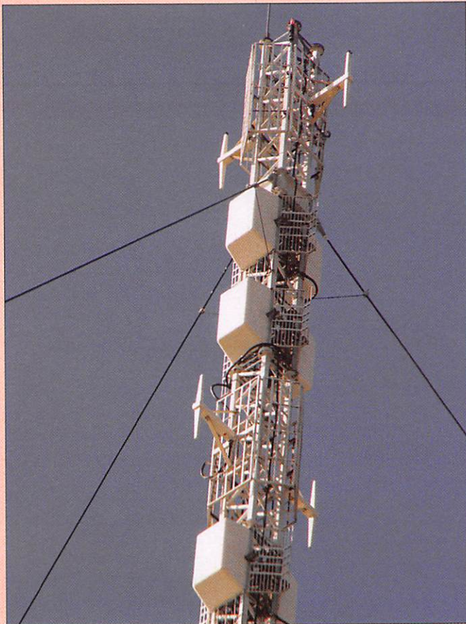
4 - Pour chaque fréquence d'émission, deux antennes panneau, placées dos à dos, assurent une couverture de 360 degrés.
