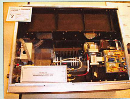
5 - Transverter 70/3 cm, 50 W HF, par F5BUU.
