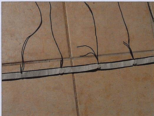
6 - Vue la boucle de finition avant mise sous tension.
